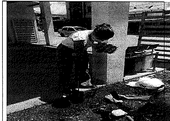
Reposición de pavimento en concreto de 4.000 Psi
